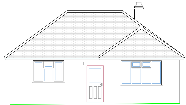
Elevation 1 Datum: 22.00m
