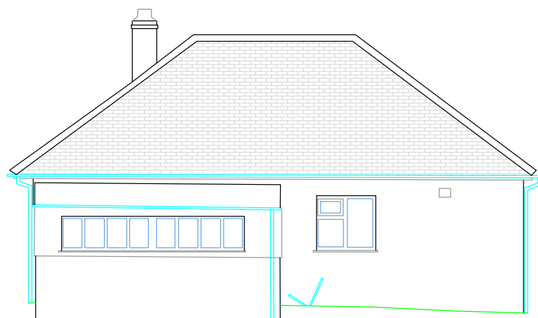
Elevation 3 Datum: 22.00m
