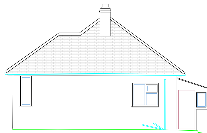
Elevation 4 Datum: 22.00m
