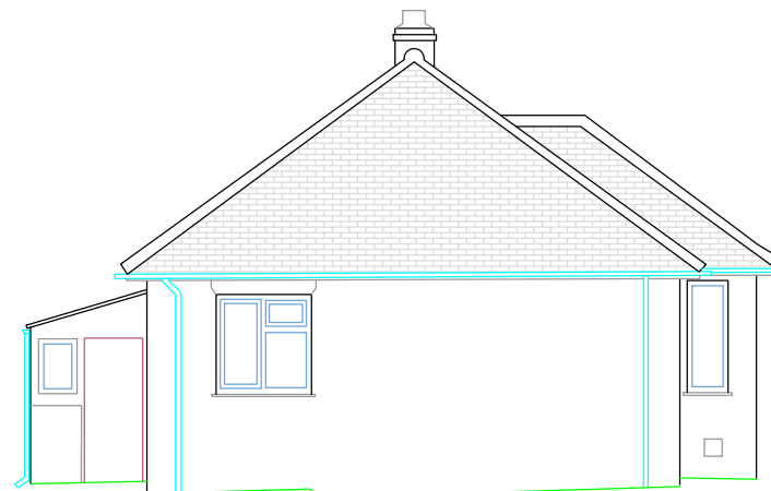
Elevation 2 Datum: 22.00m
