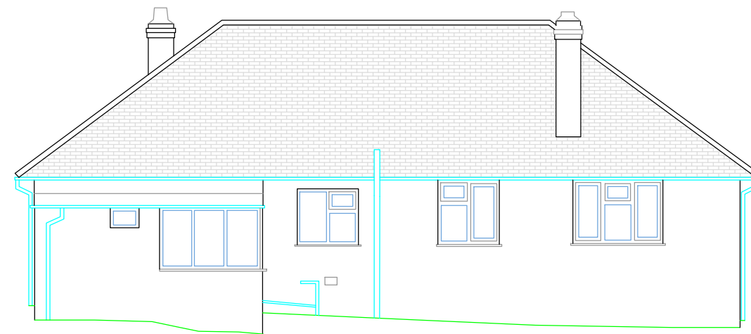
Elevation 4 Datum: 22.00m
