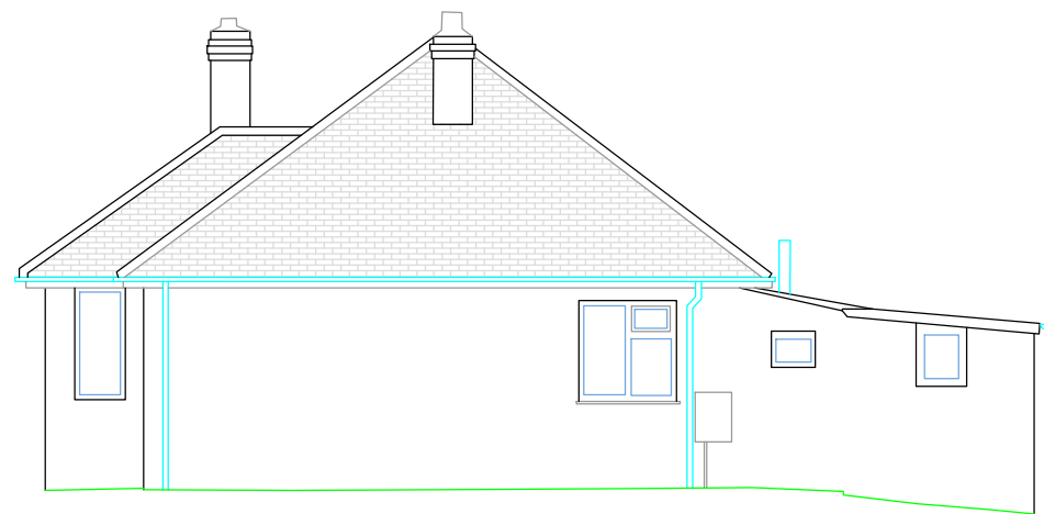
Elevation 3 Datum: 22.00m
