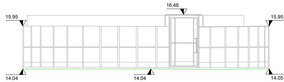
Elevation 5 Datum: 12.00m
